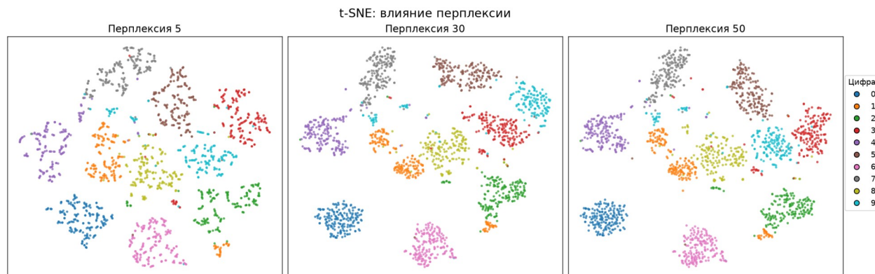
Рис. 4. t-SNE при разных значениях перплексии
